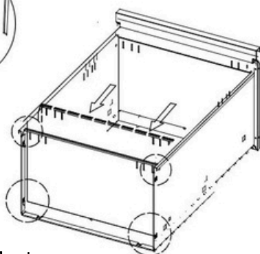
Montera lådans frontpanel enligt bilden.
