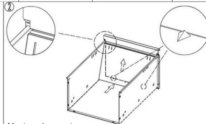
Monteer de voorste ladeafdichting zoals weergegeven op de afbeelding.
