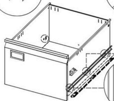
Monte las guías interiores.
