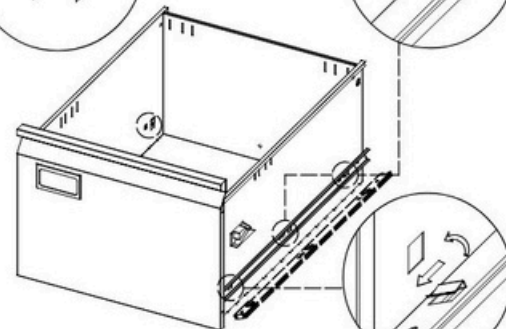
Nainštalujte vnútorné kolajnice.
