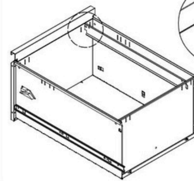
Fastgør ophængsstængerne til skuffepanelerne som vist på billedet.
