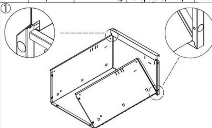
Ράβδος κλειδώματος: 1 τεμ.
