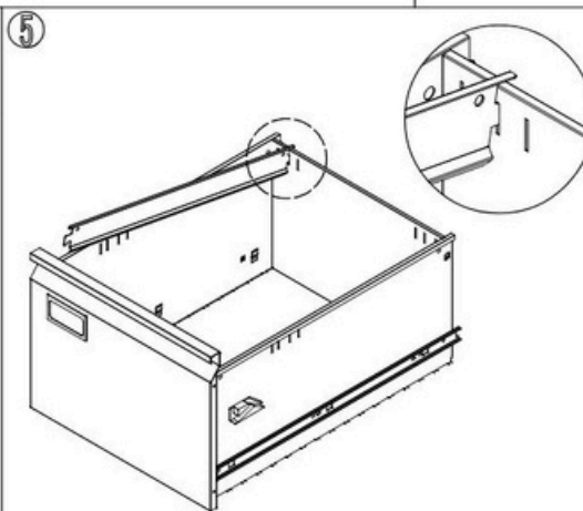
Asenna ripustustangot.
