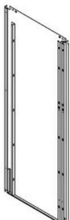
Prawa strona: 1 szt.
