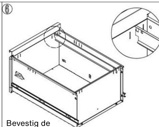
Monteer de voorste ladeafdichting zoals weergegeven op de afbeelding.
