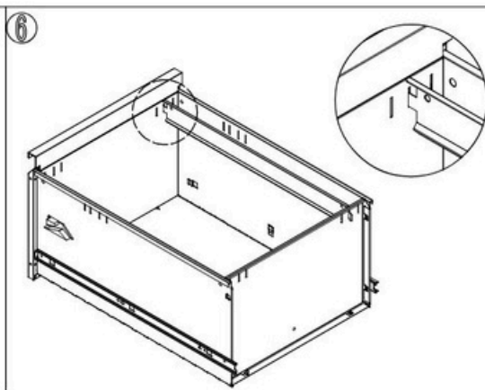
Pričvrstite šipke za kačenje na panele fioke kao što je prikazano na slici.
