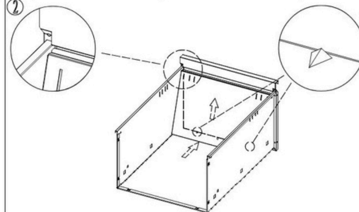
Montera den främre lådtätningen enligt bilden.
