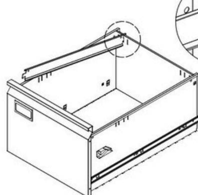
Szerelje fel a függesztőrudakat.
