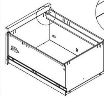
Rögzítse a függesztőrudakat a fiókelőlapokhoz az ábrának megfelelően.
