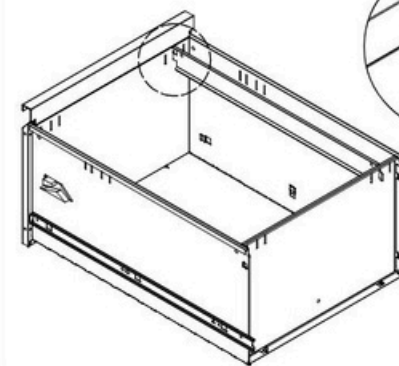
Fixați barele de suspendare pe panourile sertarelor conform imaginii.
