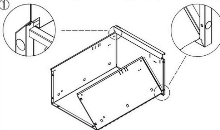
Montera den vikbara låddboxen.
