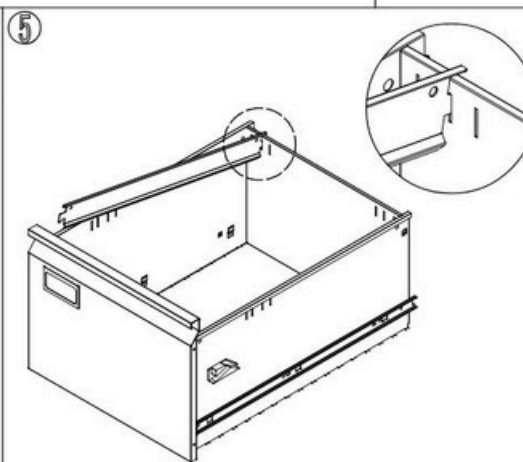
Τοποθετήστε τις ράβδους ανάρτησης.
