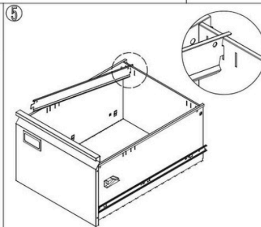
Встановіть штанги для підвішування.
