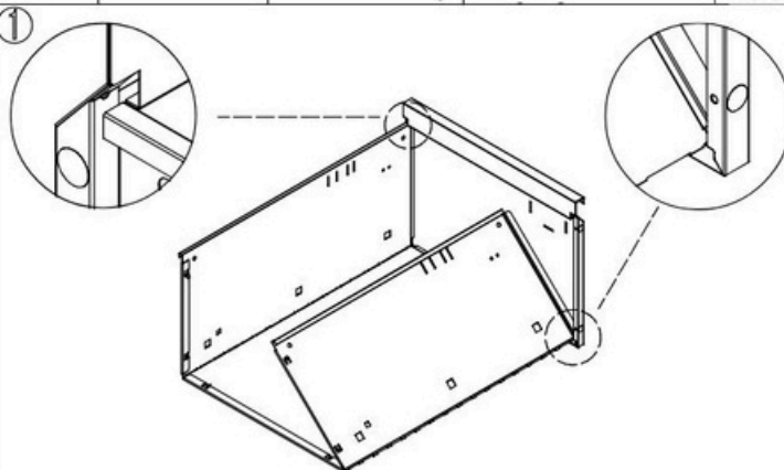
Встановіть складаний шухлядний короб.
