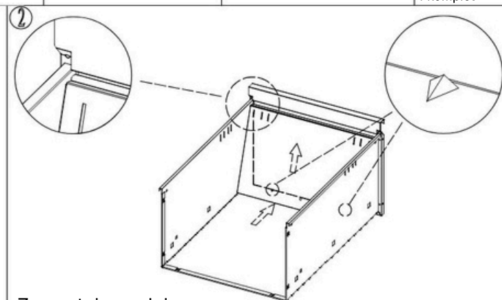
Zamontuj przednią uszczelkę szuflady zgodnie z rysunkiem.
