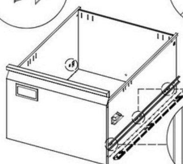
Montirajte unutarnje vodilice.
