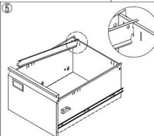
Monteer de ophangstangen.
