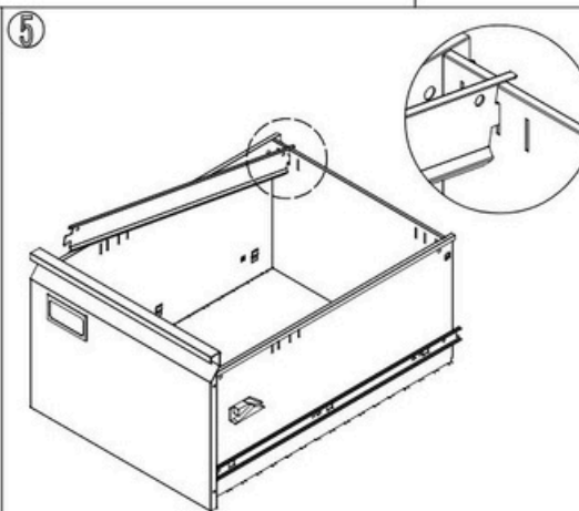
Paigaldage riputusvardad.
