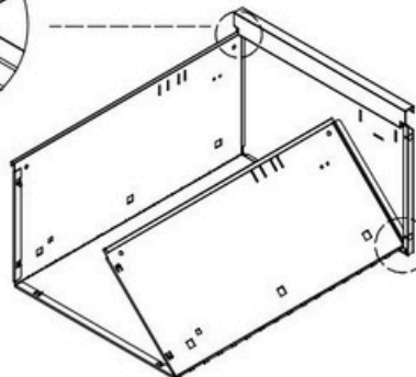
Monter den sammenleggbare skuffeboksen.
