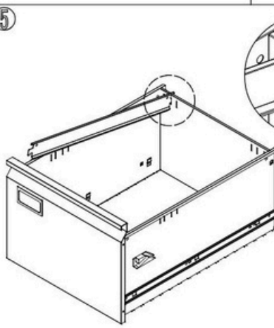
Установите штанги для подвешивания.
