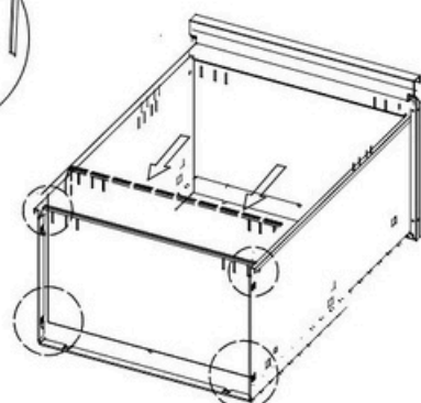
Τοποθετήστε το μπροστινό πάνελ του συρταριού όπως φαίνεται στην εικόνα.
