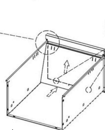
Monter den forreste skuffetætning som vist på billedet.
