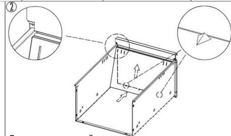
Встановіть передній ущільнювач шухляди, як показано на зображенні.
