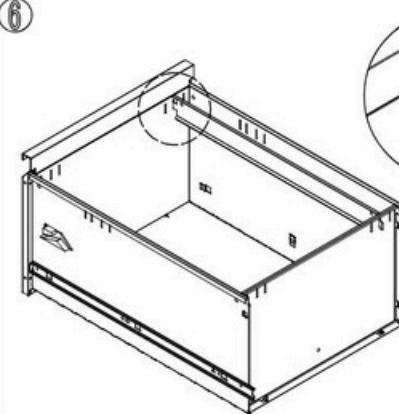
Obešalne palice pritrdite na panele predalov, kot je prikazano na sliki.
