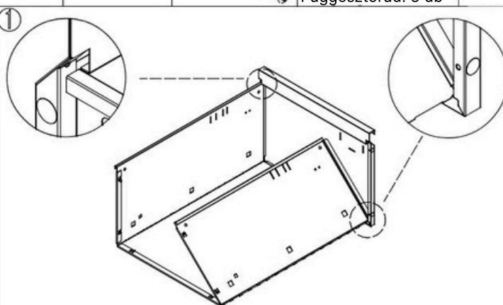
Zárórúd: 1 db
