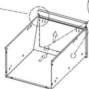
Monter den fremre skuffetetningen som vist på bildet.
