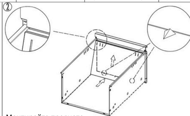
Монтирайте предното уплътнение на чекмеджето според изображението.
