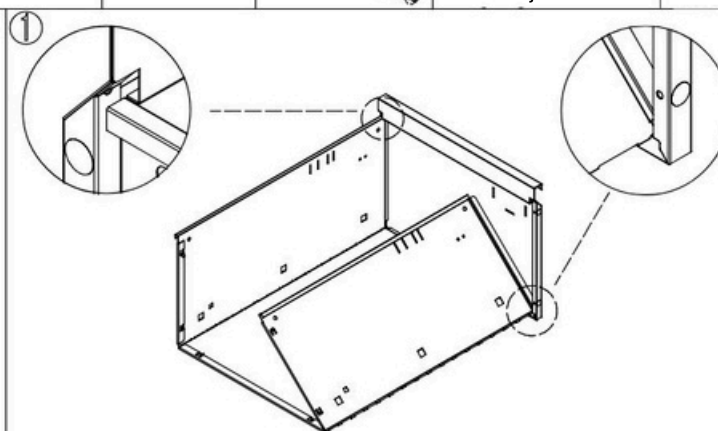
Montirajte sklopivu kutiju fioke.
