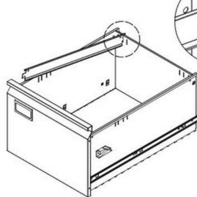
Monter opphengsstengene.
