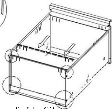
Szerelje fel a fiók előlapját az ábrának megfelelően.
