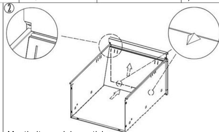
Montirajte prednju zaptivku fioke kao što je prikazano na slici.
