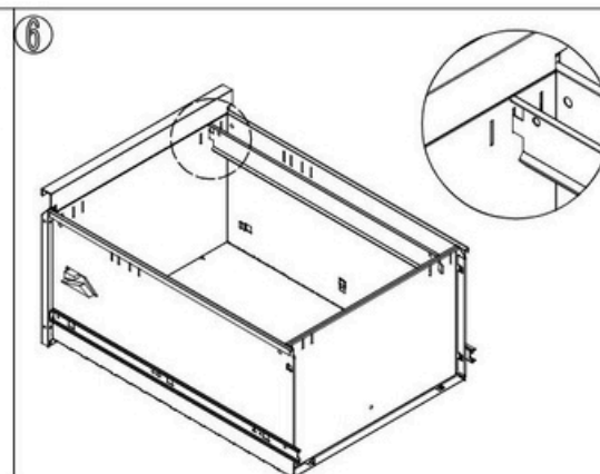
Přípevněte závěsné tyče k panelům zásuvek podle obrázku.
