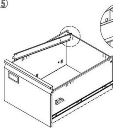
Monte las barras de suspensión.
