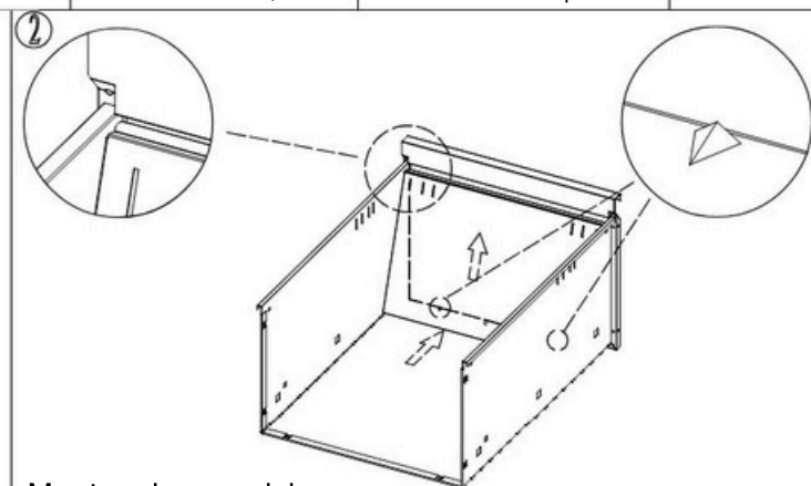
Montare la guarnizione anteriore del cassetto come mostrato nell'immagine.
