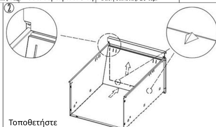
Κουτί συρταριού: 5 τεμ.
