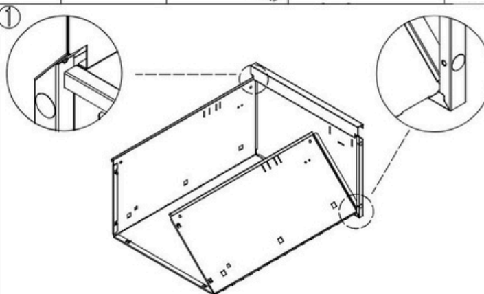
Monte la caja plegable del cajón.
