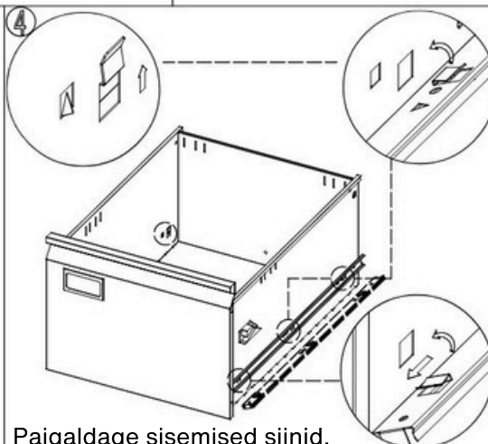
Paigaldage sisemised siinid.
