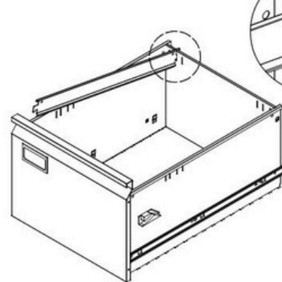
Montera upphängningsstängerna.
