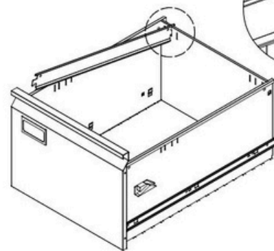
Montați barele de suspendare.
